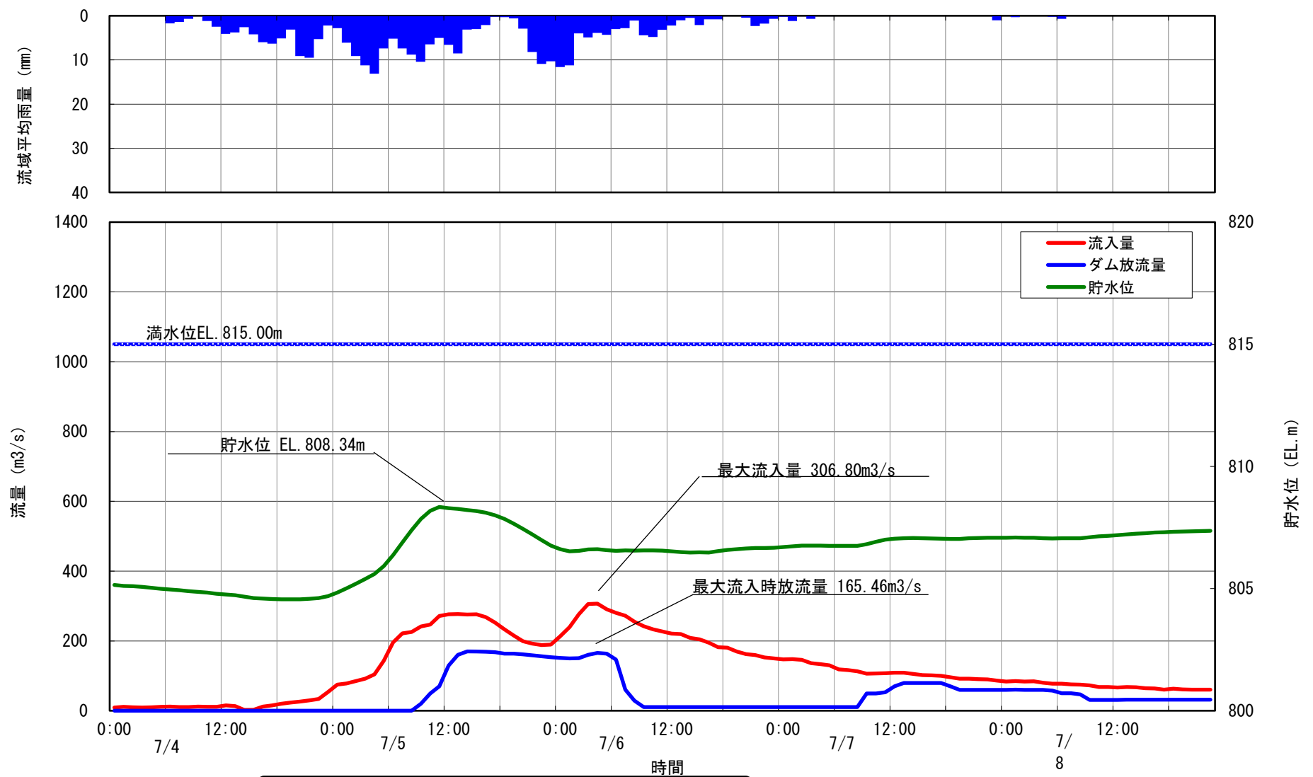
24 美和ダム洪水調節図 平成30年7月6日洪水
