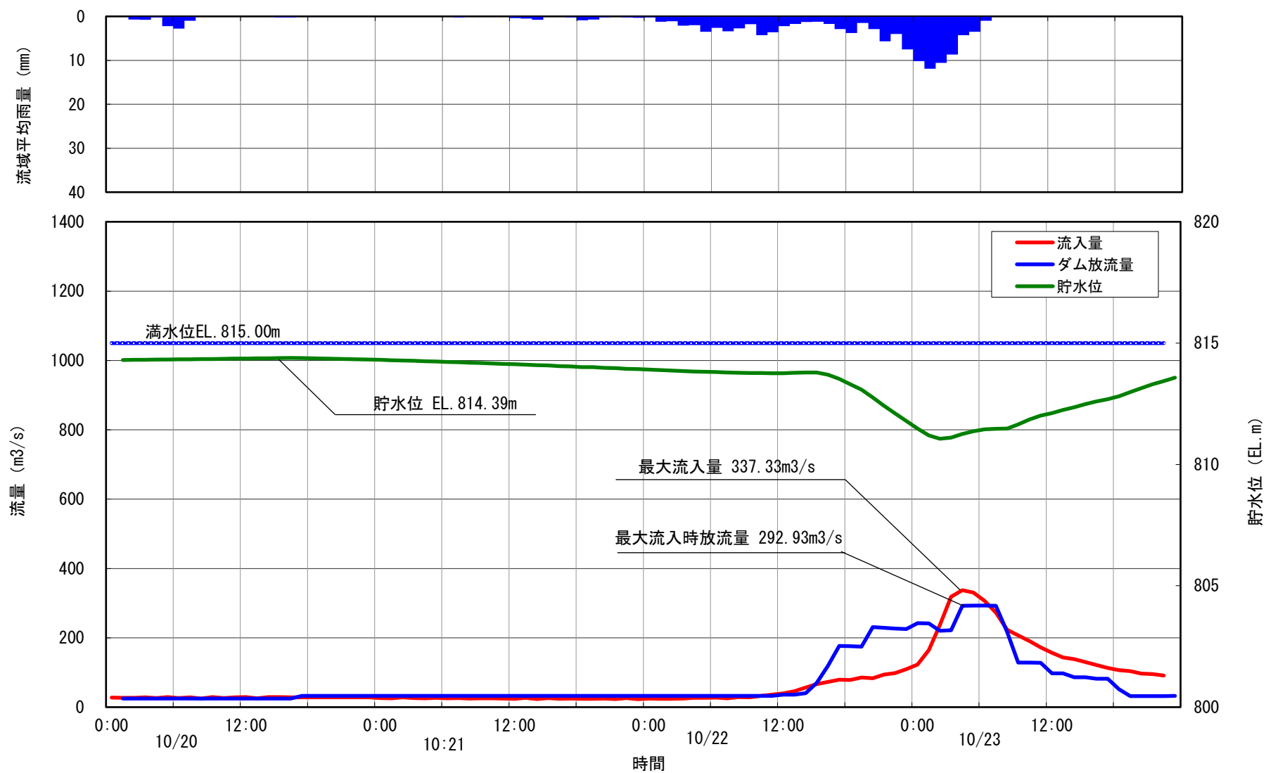
23 美和ダム洪水調節図 平成29年10月23日洪水
