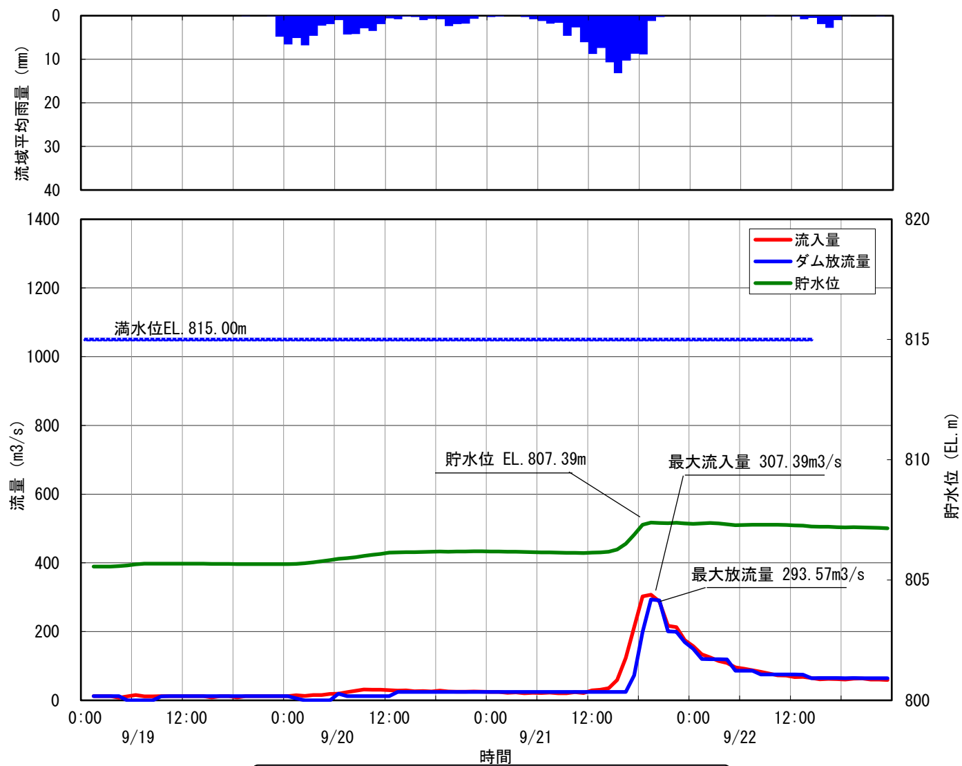
22 美和ダム洪水調節図 平成23年9月21日洪水
