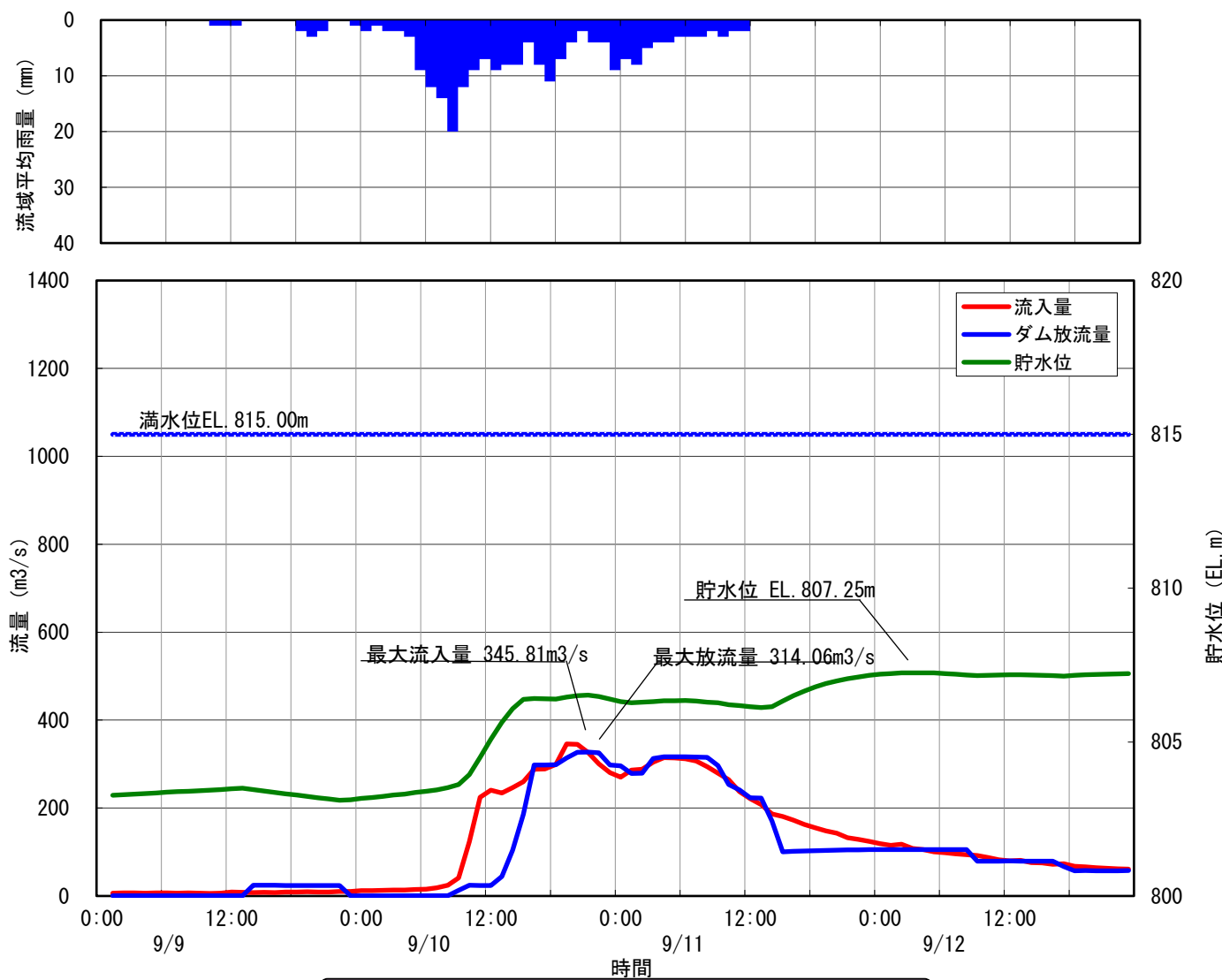
18 美和ダム洪水調節図 平成13年9月10日洪水
