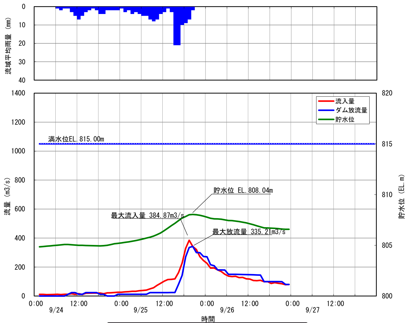
17 美和ダム洪水調節図 昭和63年9月25日洪水
