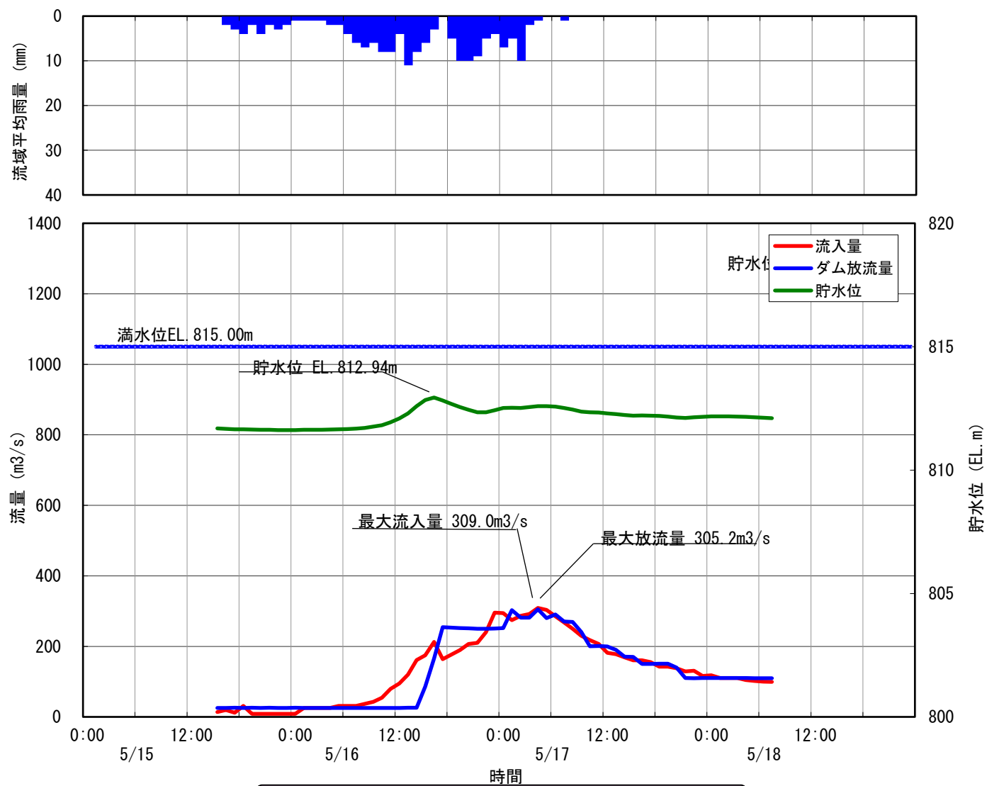
13 美和ダム洪水調節図 昭和58年5月17日洪水
