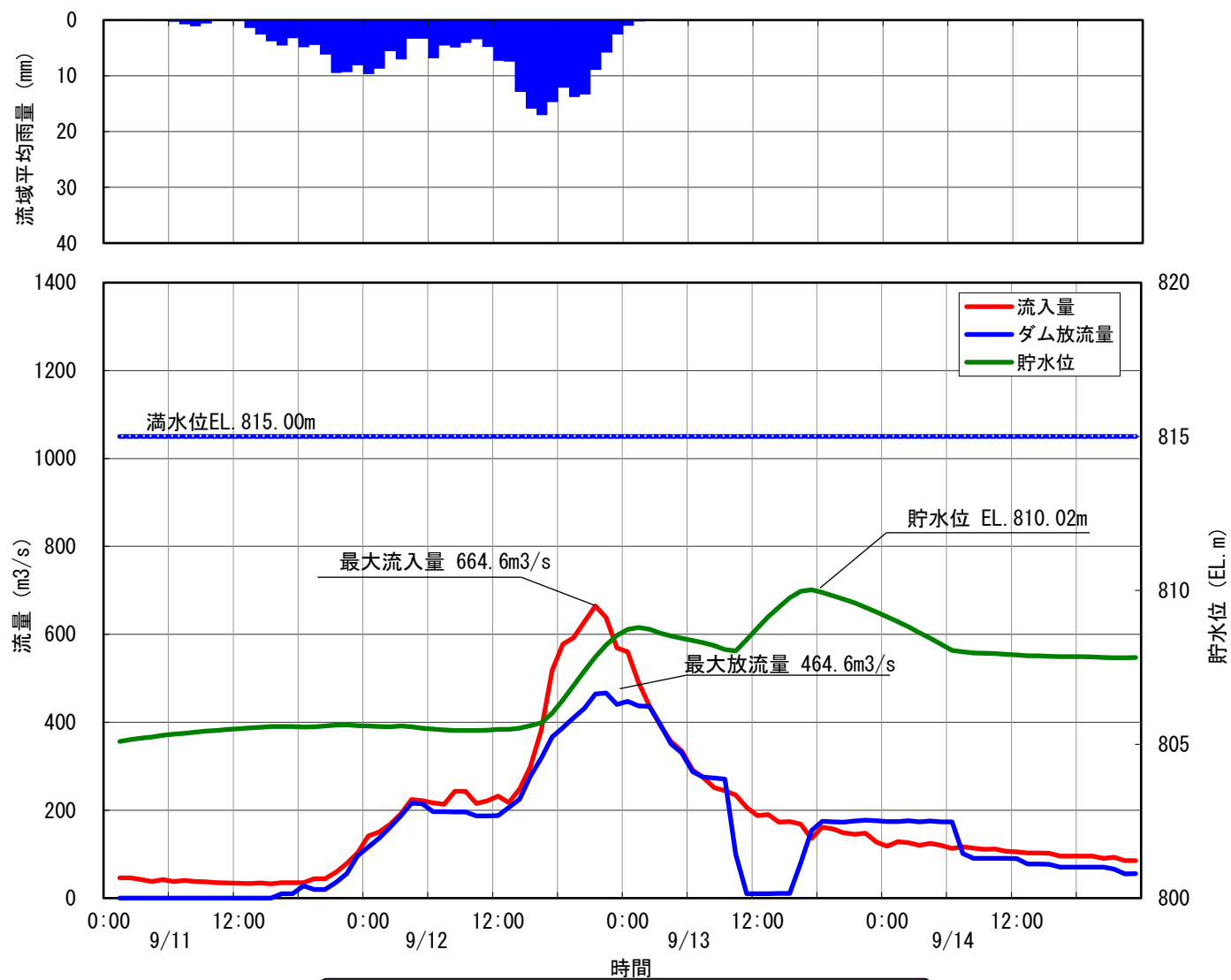
12 美和ダム洪水調節図 昭和57年9月12日洪水
