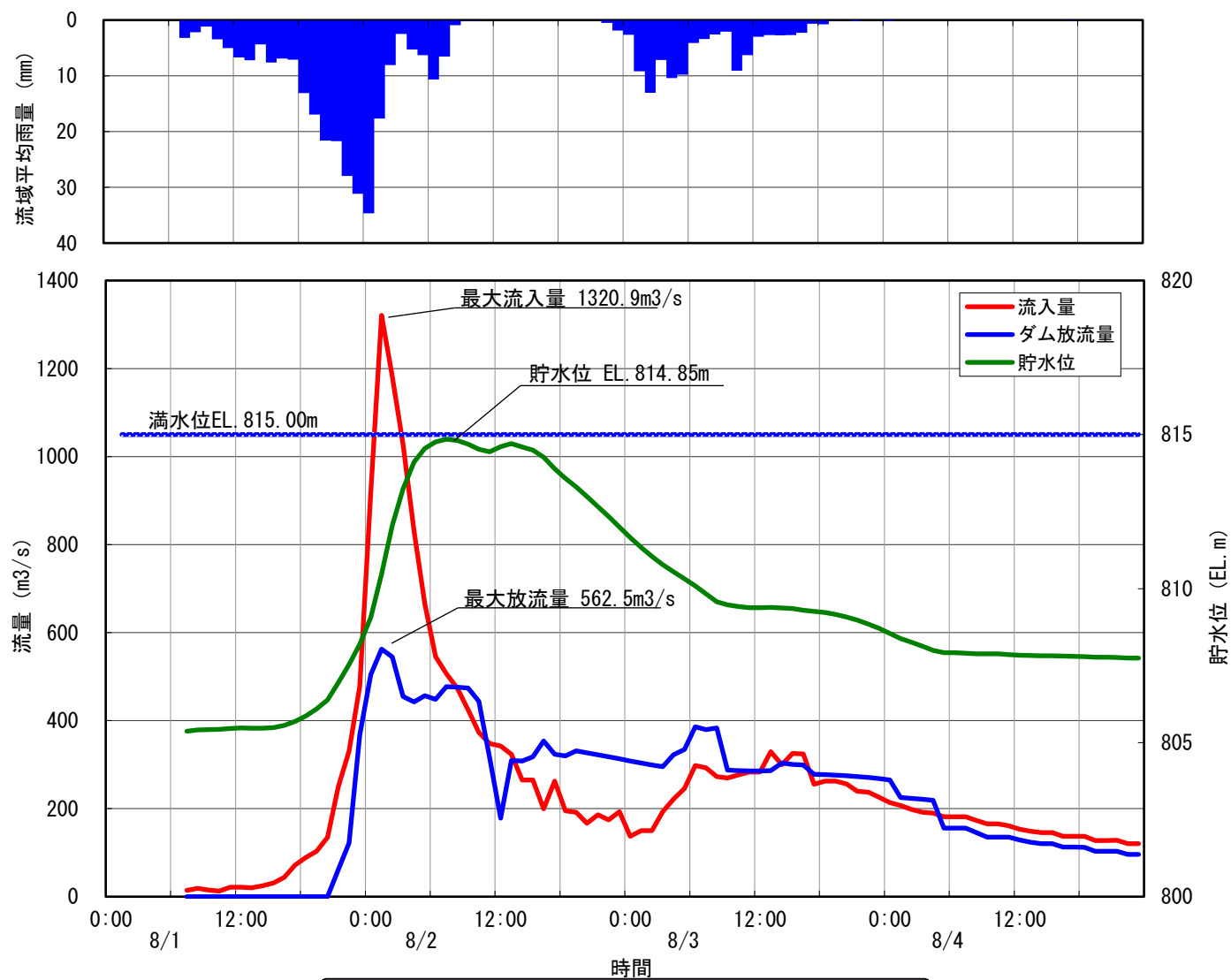
11 美和ダム洪水調節図 昭和57年8月1日洪水
