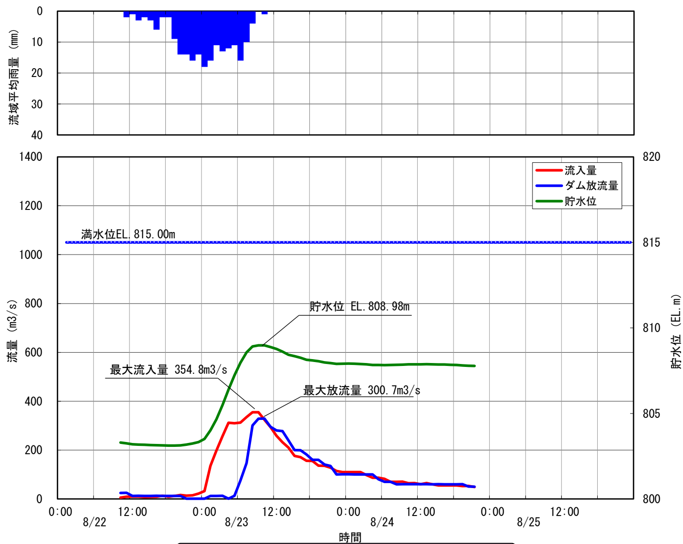
10 美和ダム洪水調節図 昭和56年8月23日洪水
