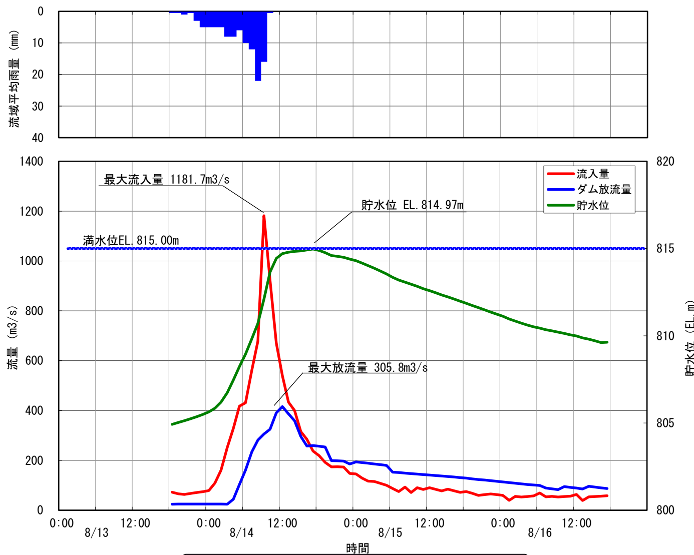
3 美和ダム洪水調節図 昭和34年8月14日洪水
