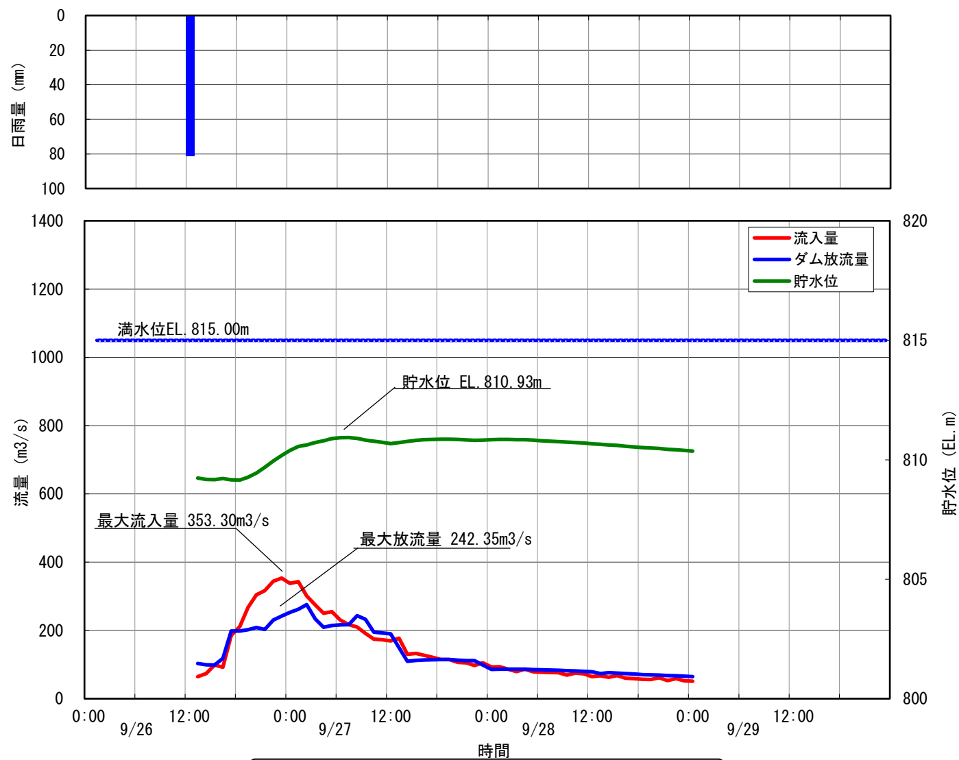
2 美和ダム洪水調節図 昭和33年9月26日洪水
