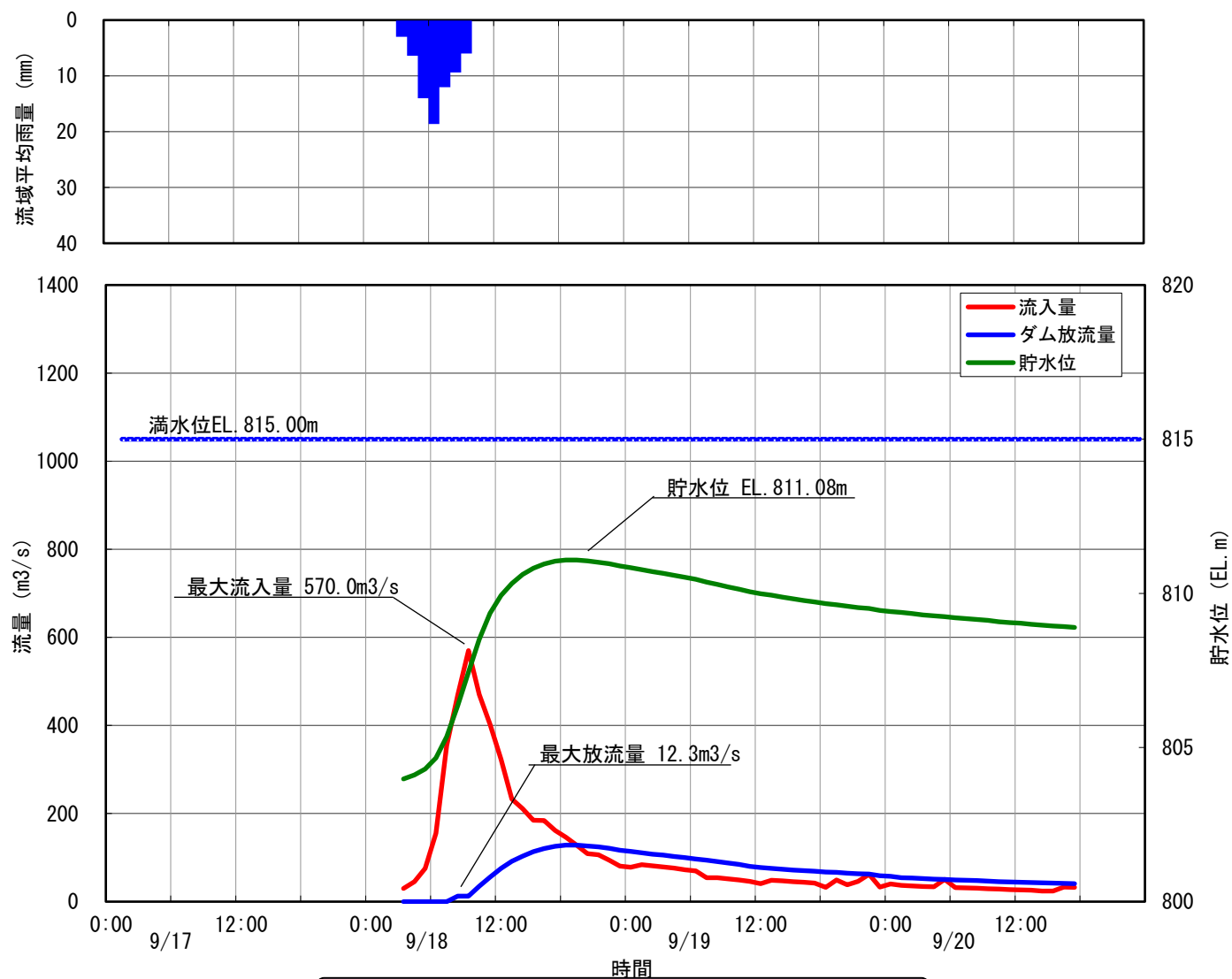
1 美和ダム洪水調節図 昭和33年9月18日洪水
