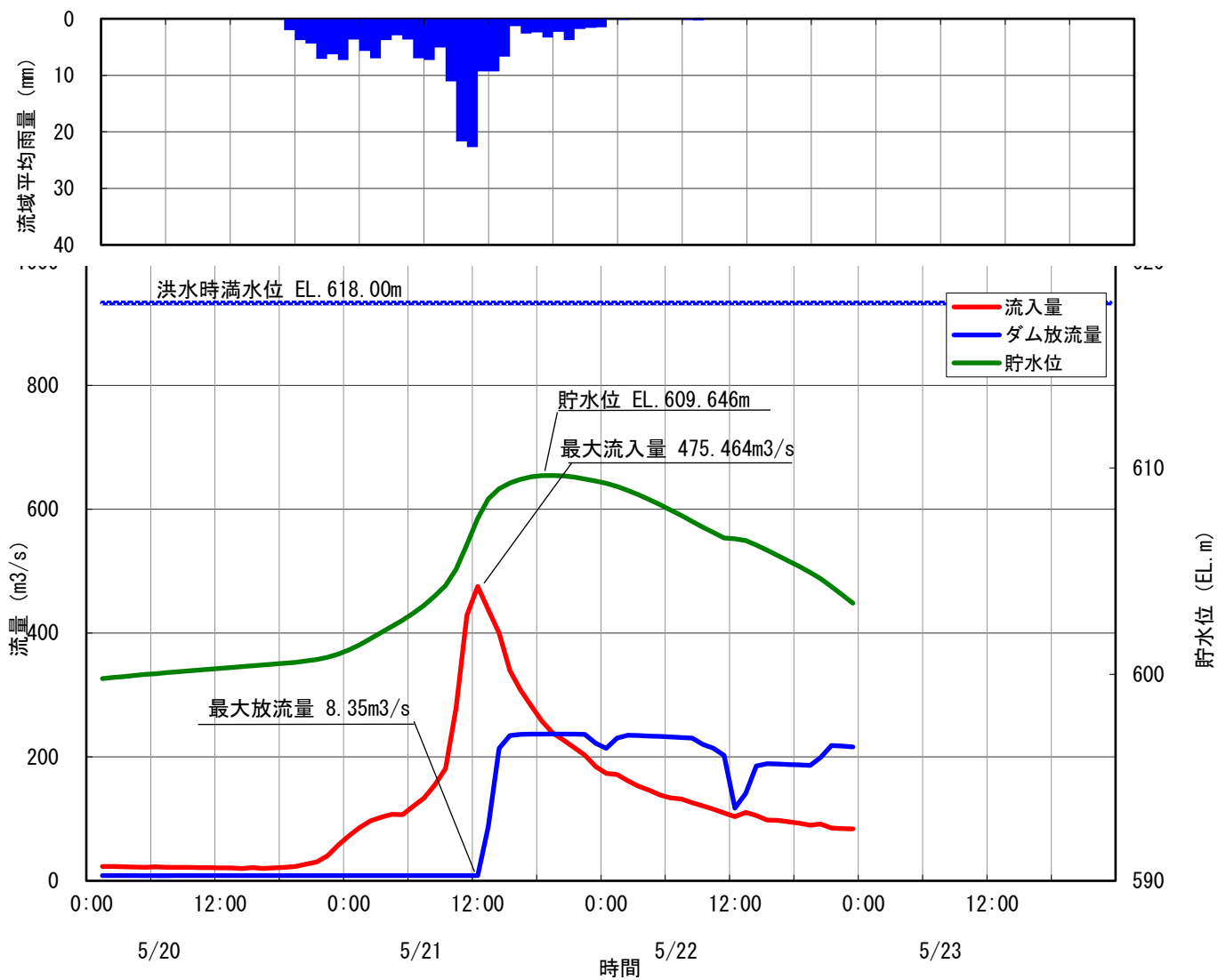
60 小渋ダム洪水調節図 令和3年 5月 21日梅雨及び低気圧
