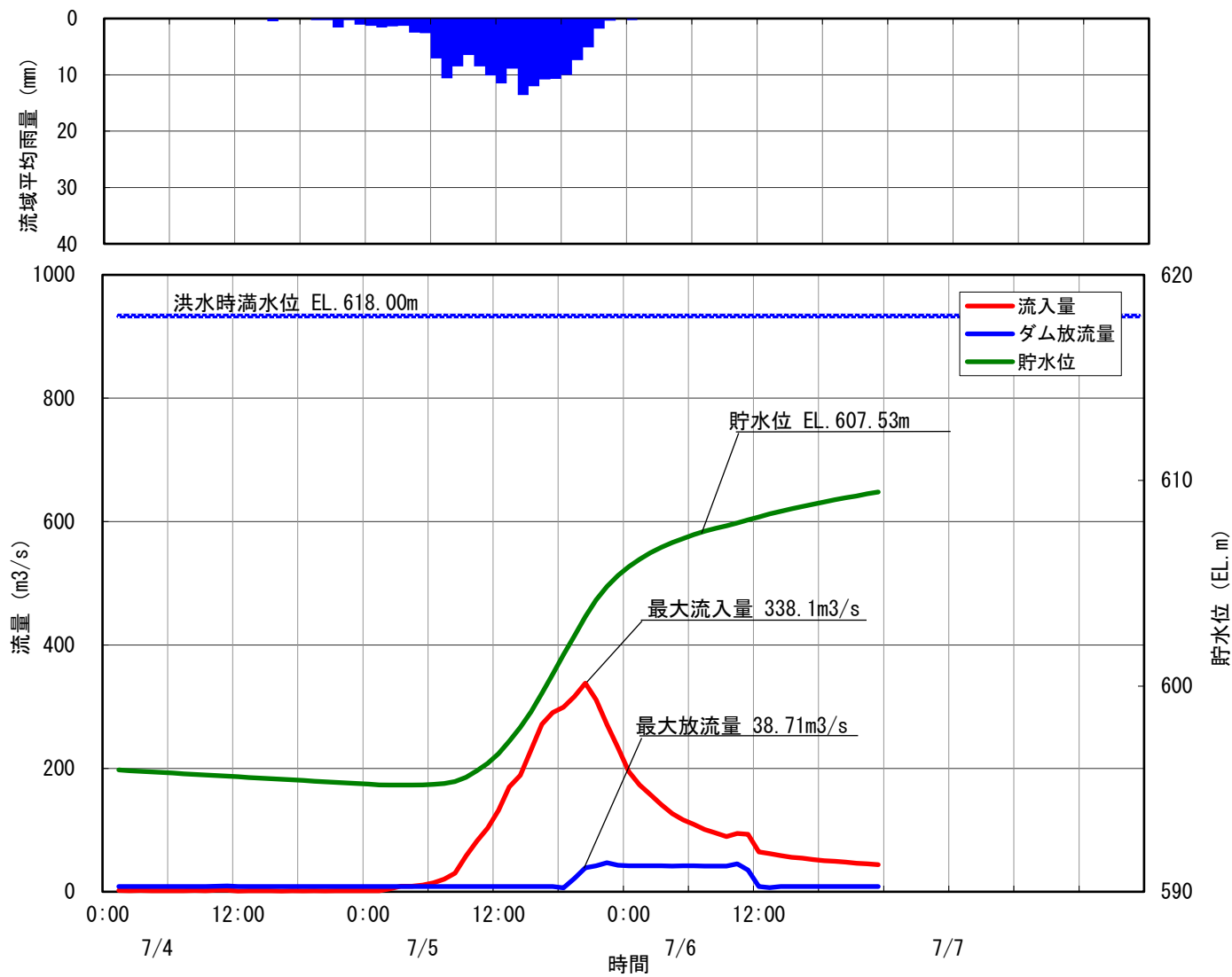
52 小洪ダム洪水調節図 令和1年10月12日19号台風
