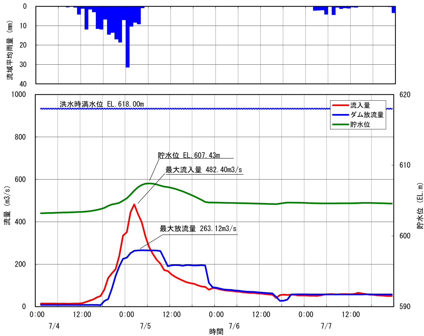
49 小渋ダム洪水調節図 平成30年9月4日台風24号
