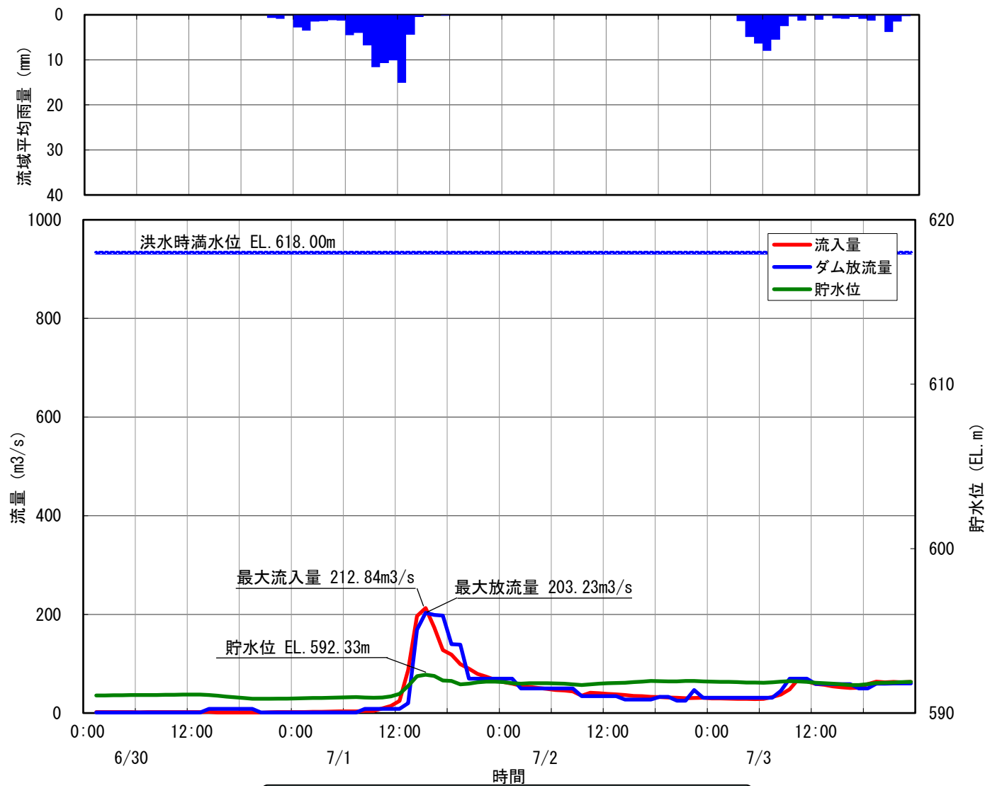
46 小渋ダム洪水調節図 平成27年7月1日洪水
