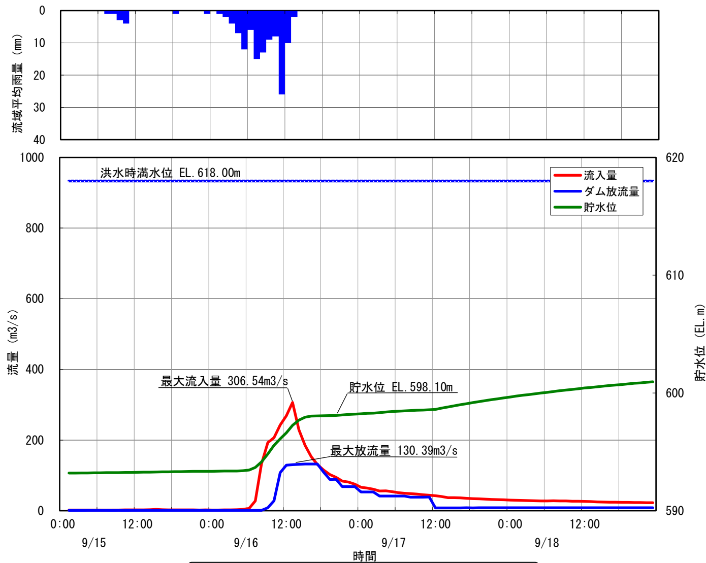
45 小渋ダム洪水調節図 平成25年9月16日洪水
