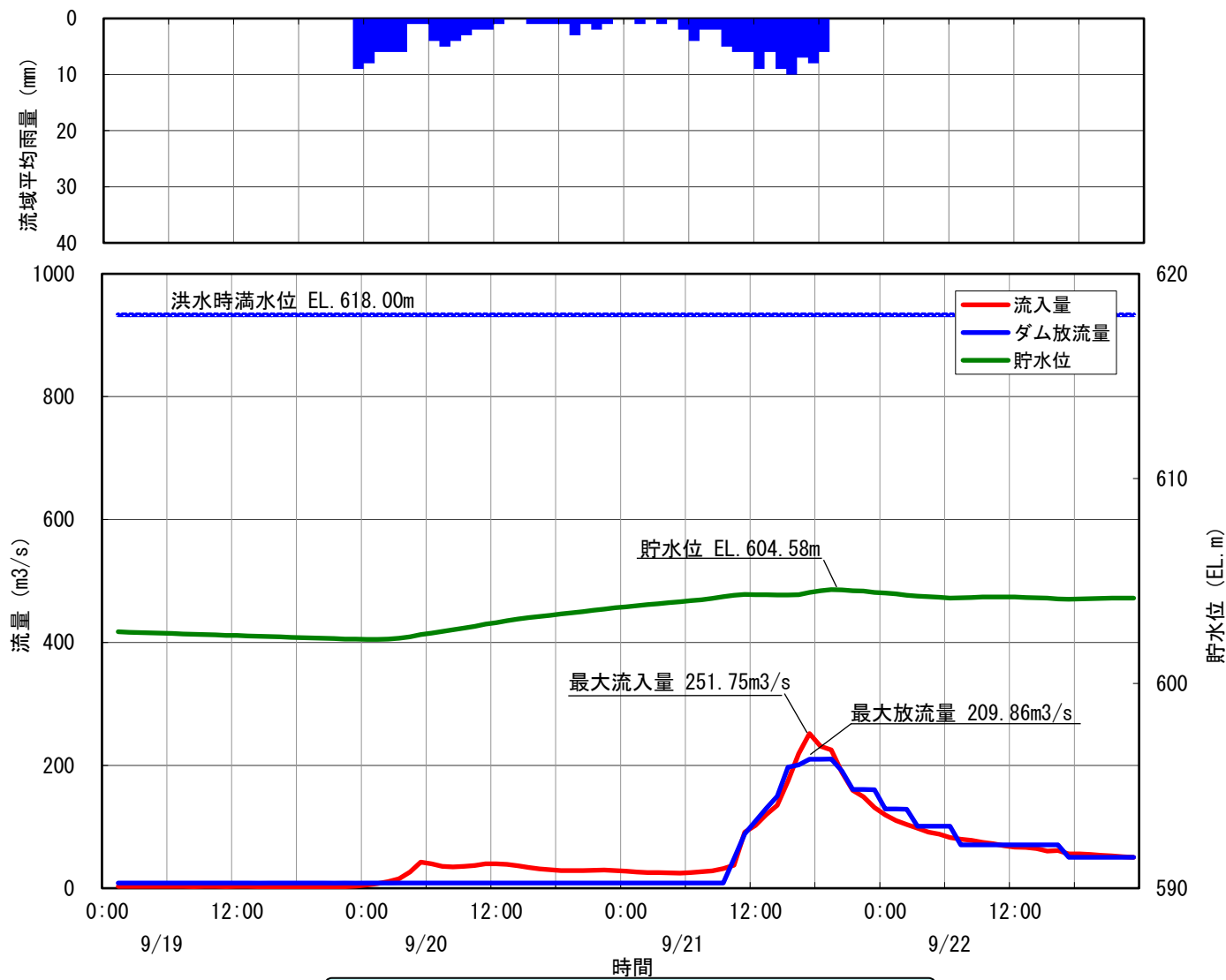
44 小渋ダム洪水調節図 平成23年9月21日洪水
