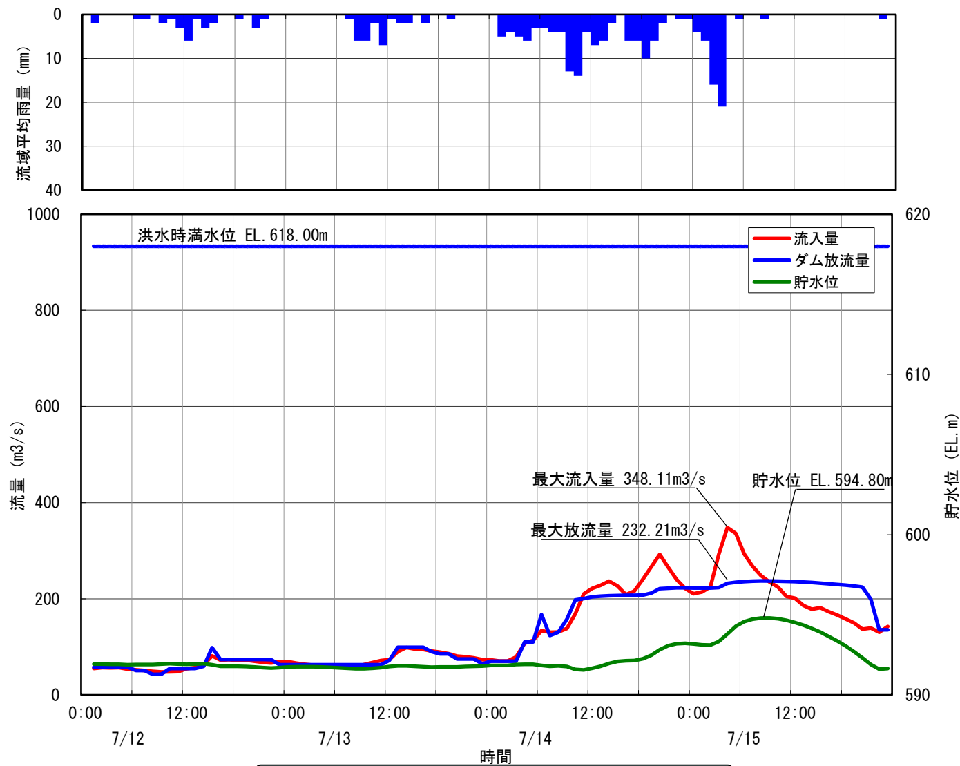
42 小渋ダム洪水調節図 平成22年7月14日洪水
