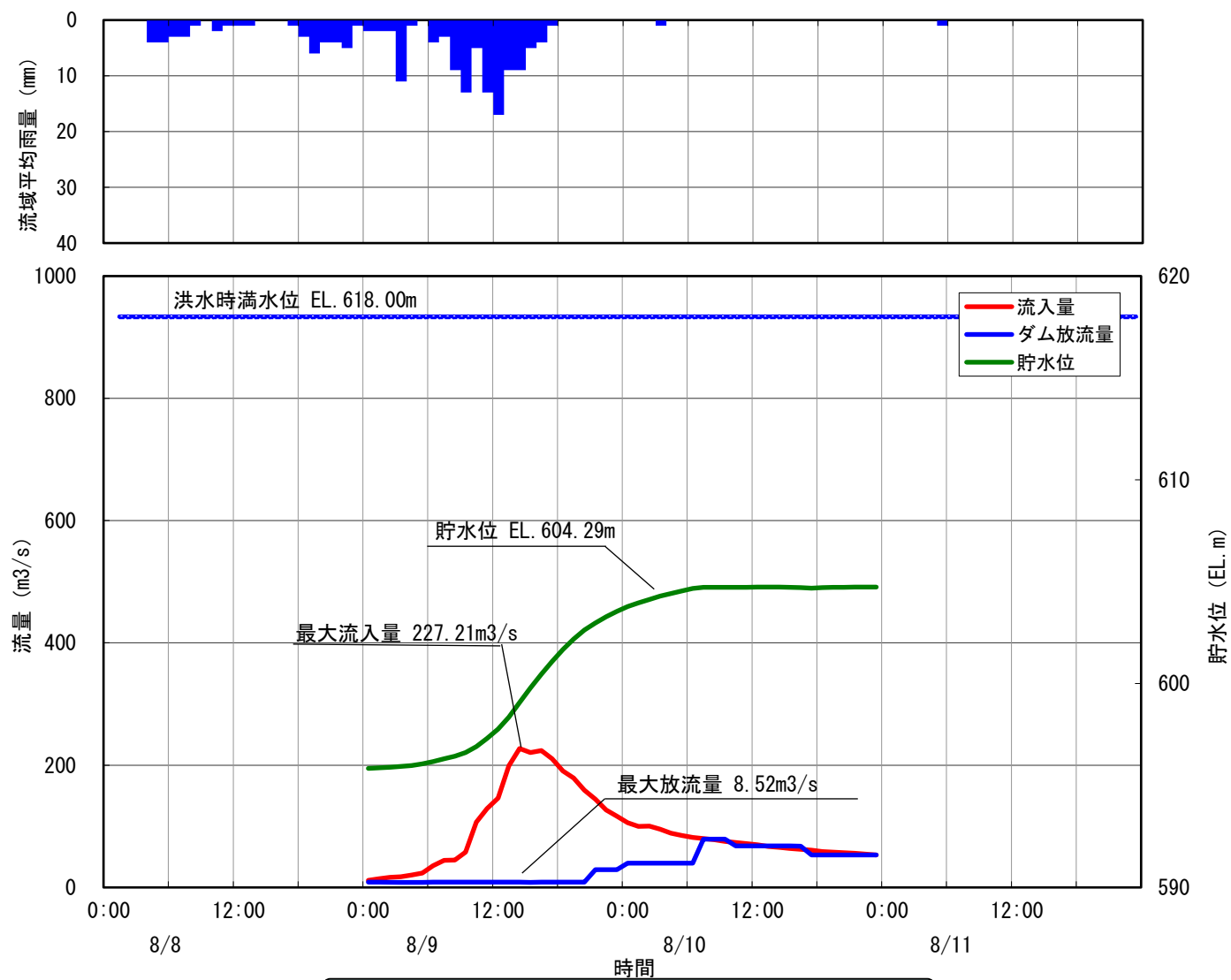
37 小渋ダム洪水調節図 平成15年8月9日洪水
