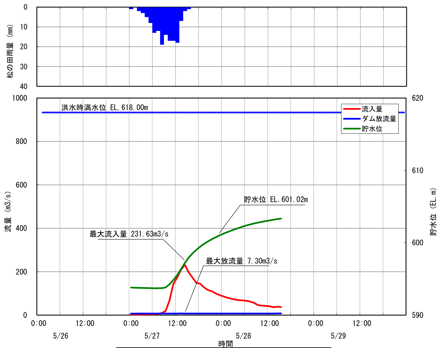
31 小渋ダム洪水調節図 平成11年5月27日洪水
