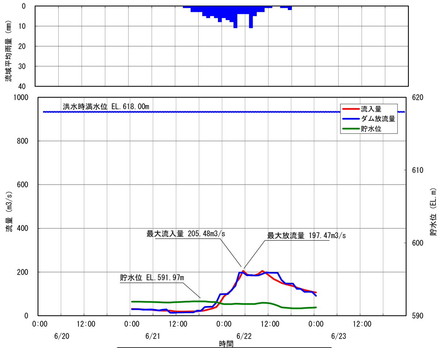
30 小渋ダム洪水調節図 平成10年6月22日洪水
