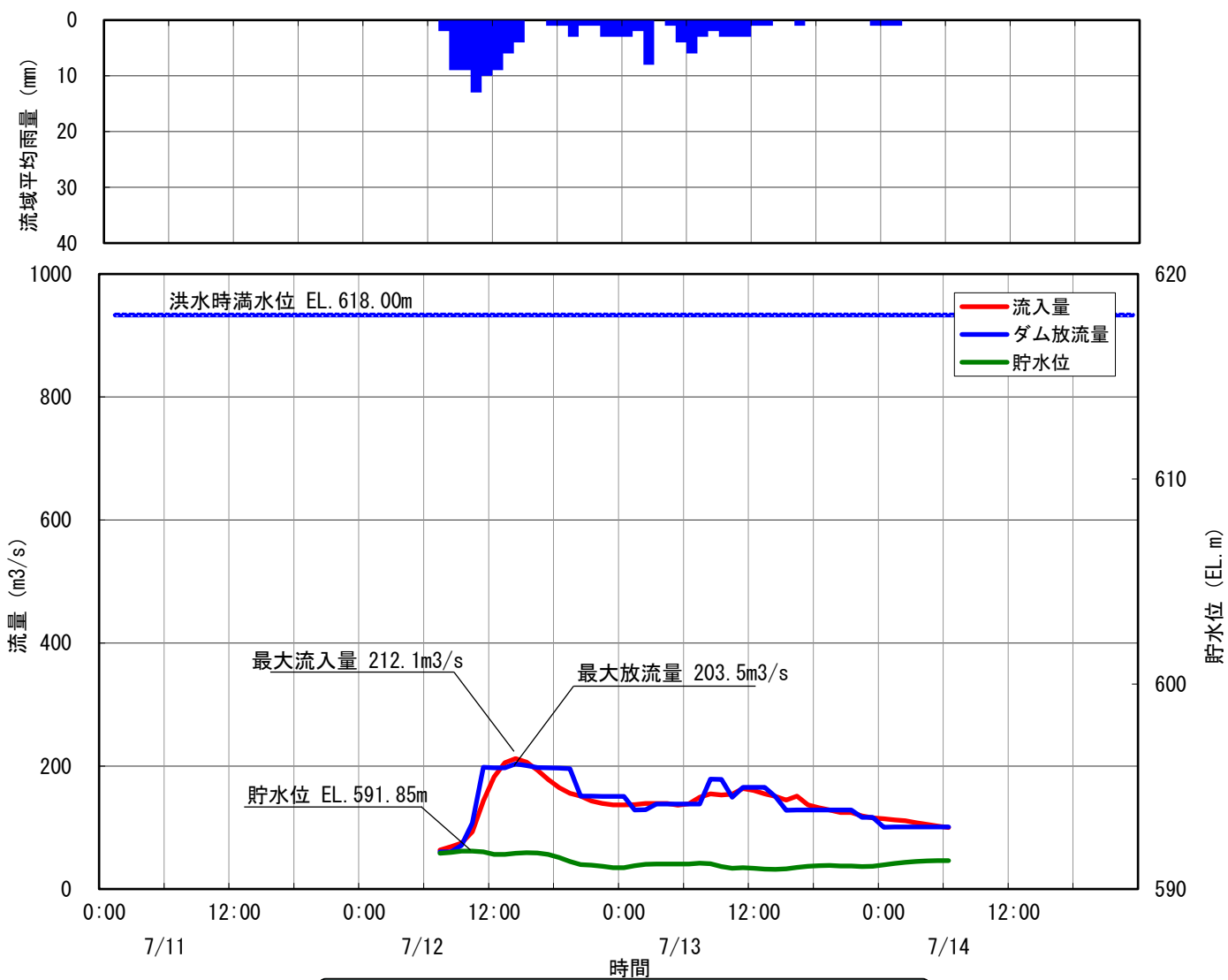
28 小渋ダム洪水調節図 平成9年7月12日洪水
