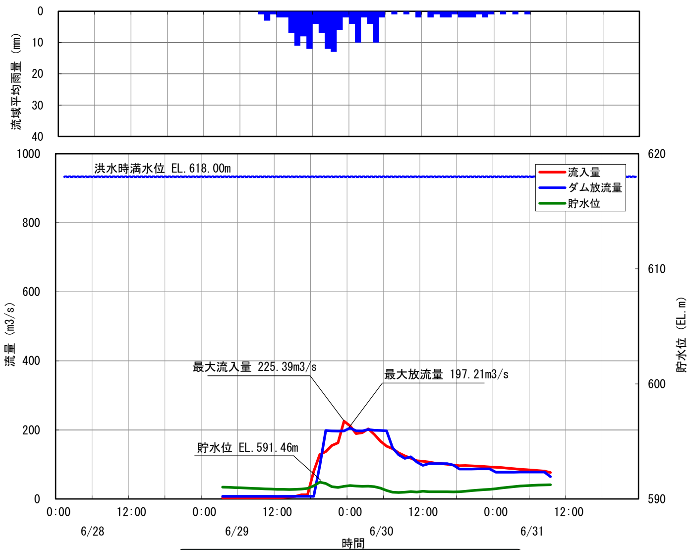
27 小渋ダム洪水調節図 平成 5年6月29日洪水
