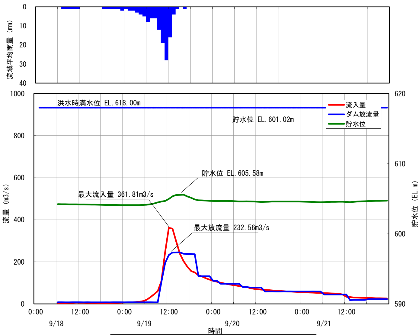
26 小渋ダム洪水調節図 平成 3年9月19日洪水
