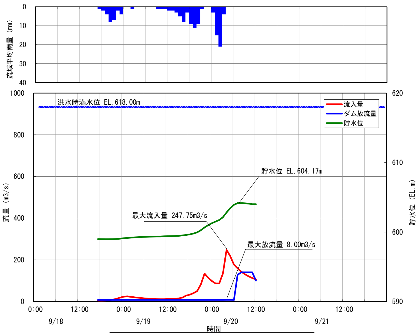
24 小渋ダム洪水調節図 平成 元年9月20日洪水
