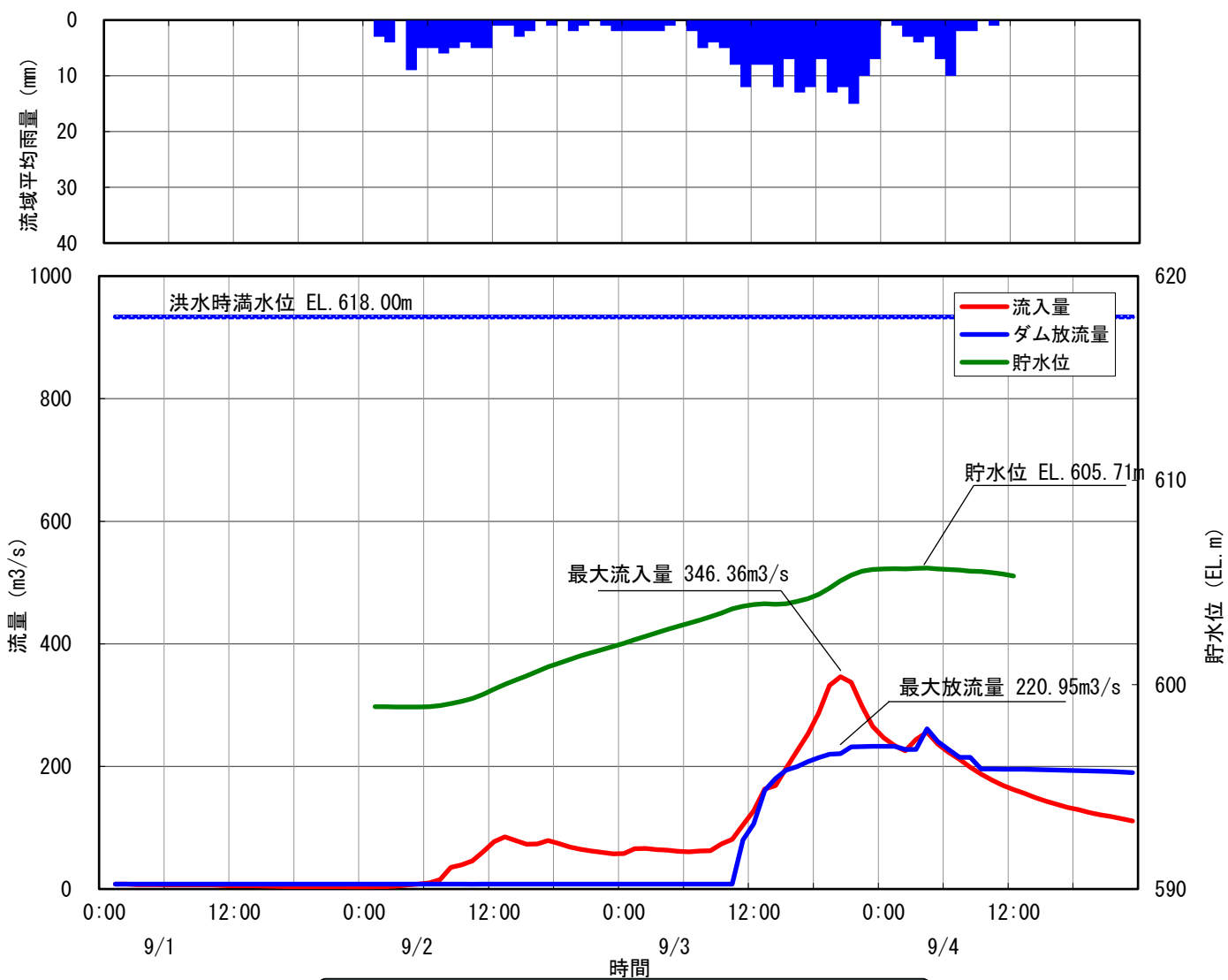
23 小渋ダム洪水調節図 平成 元年9月3日洪水
