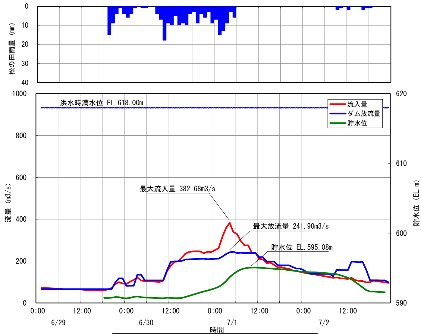
20 小渋ダム洪水調節図 昭和60年6月30日洪水
