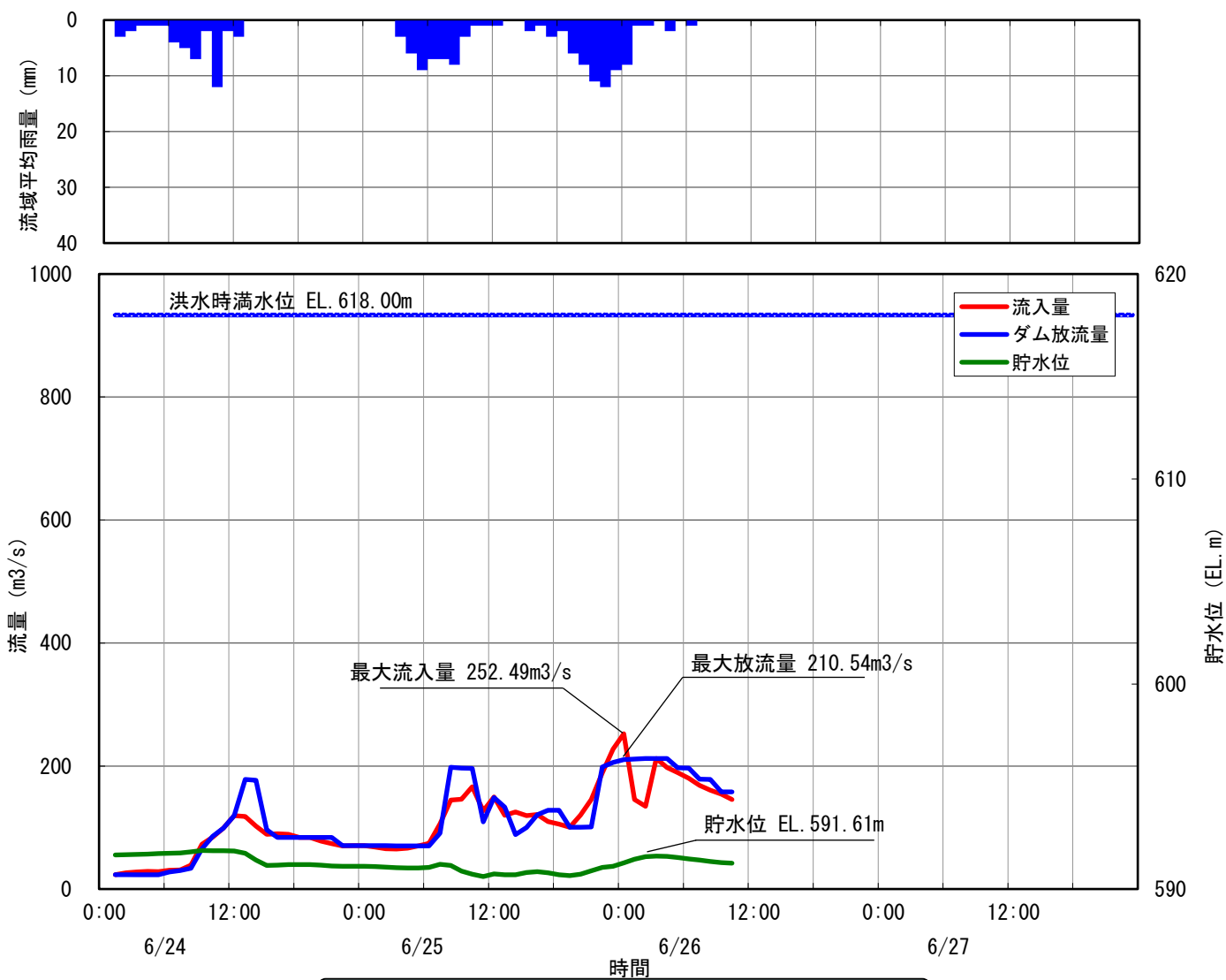
19 小渋ダム洪水調節図 昭和60年6月25日洪水
