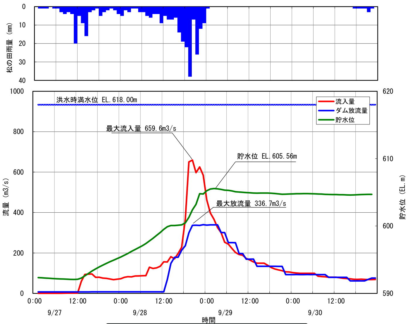
18 小渋ダム洪水調節図 昭和58年9月28日洪水
