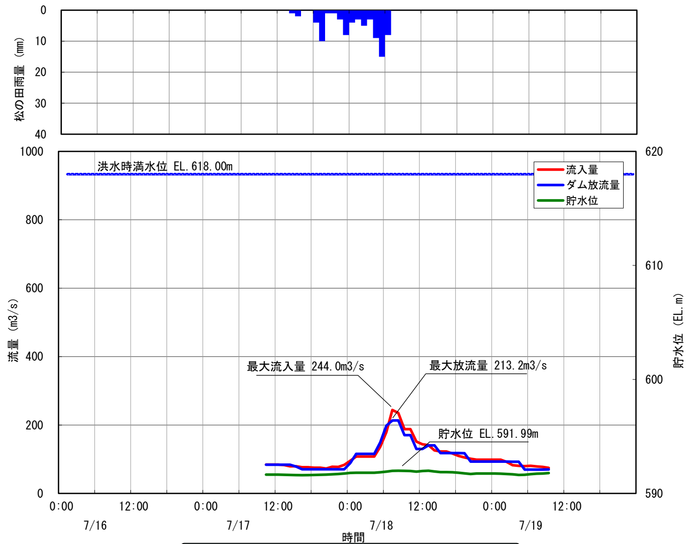
17 小渋ダム洪水調節図 昭和58年7月18日洪水
