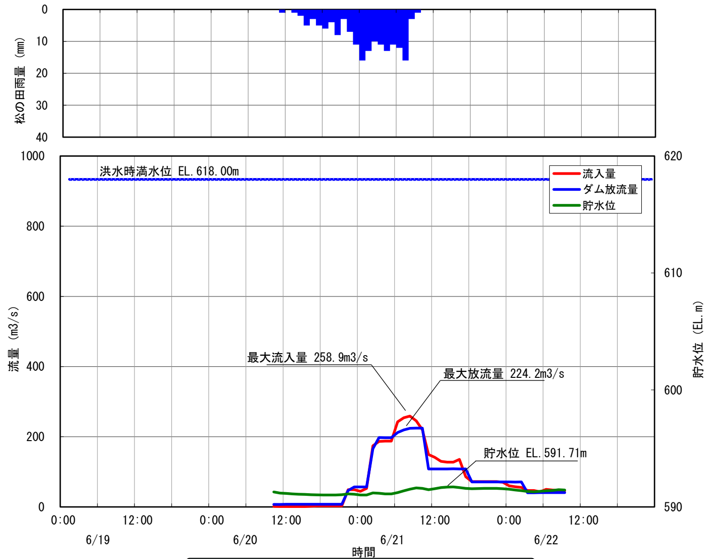
16 小渋ダム洪水調節図 昭和58年6月21日洪水
