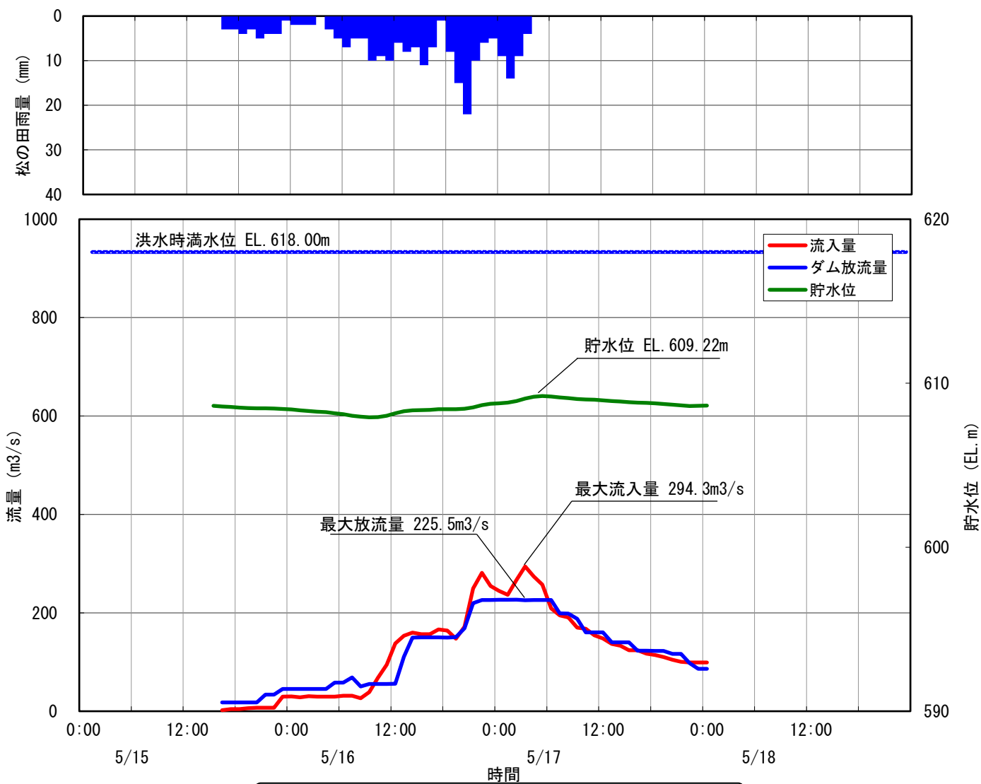
15 小渋ダム洪水調節図 昭和58年5月16日洪水
