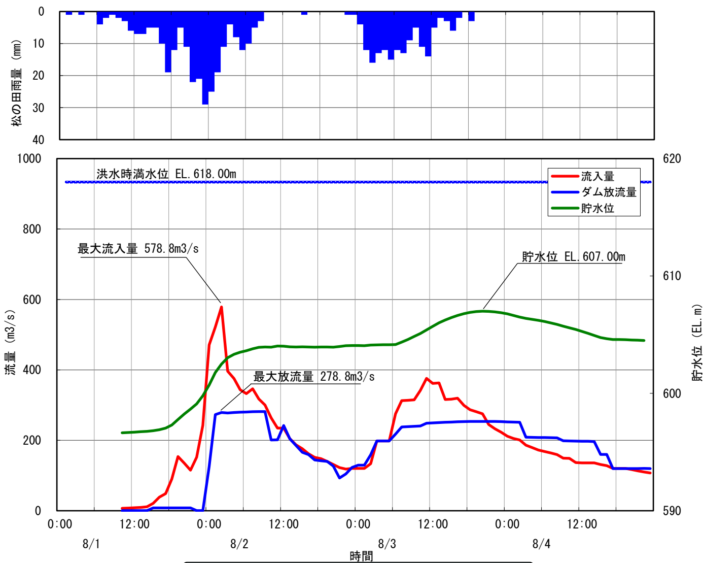
13 小渋ダム洪水調節図 昭和57年8月2日洪水
