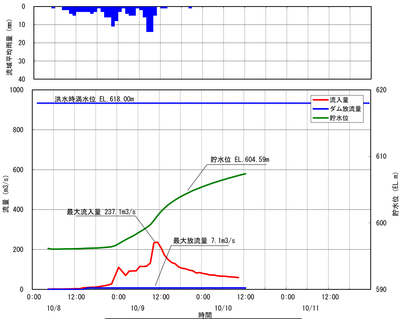
12 小渋ダム洪水調節図 昭和56年10月9日洪水
