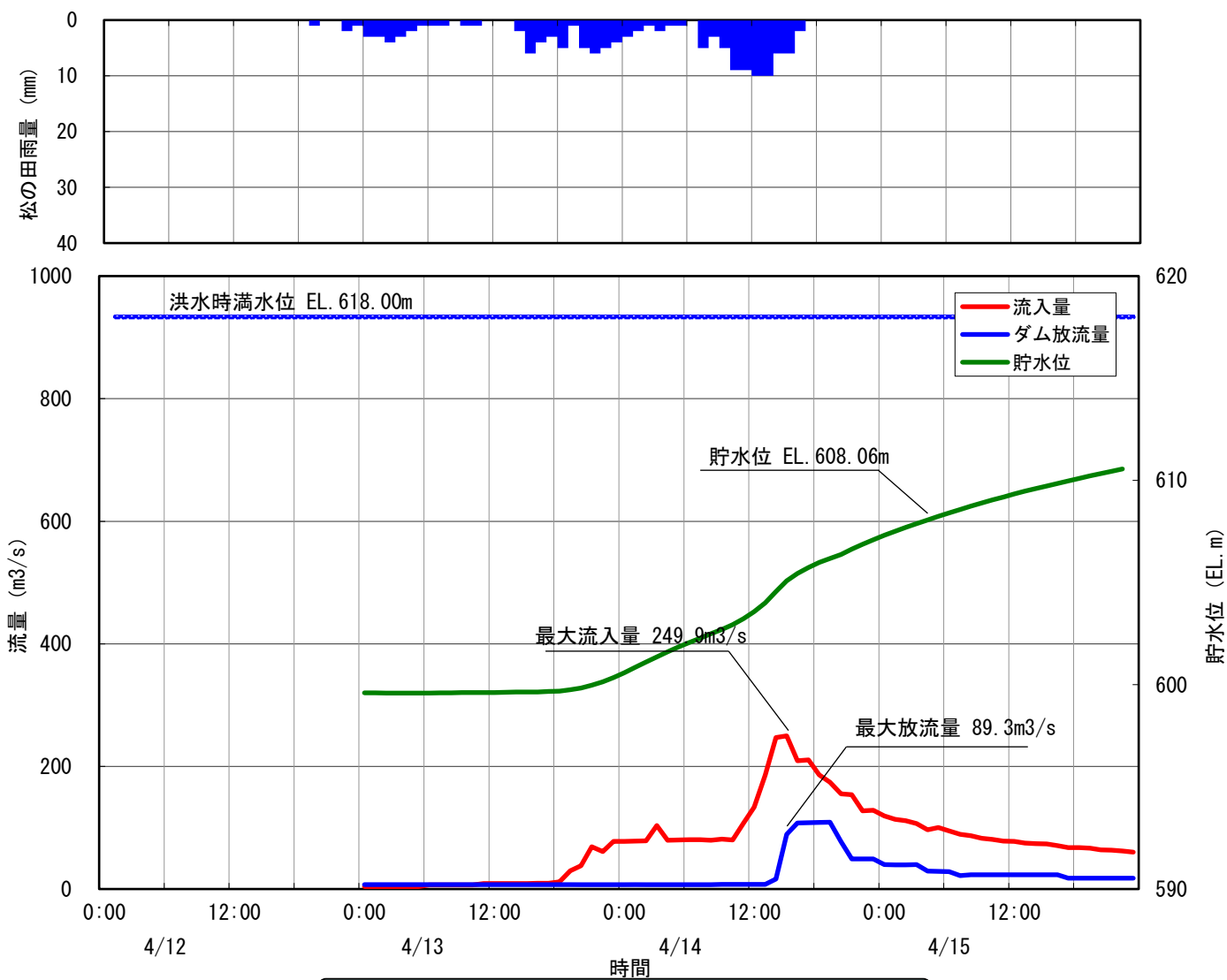
11 小渋ダム洪水調節図 昭和55年4月14日洪水
