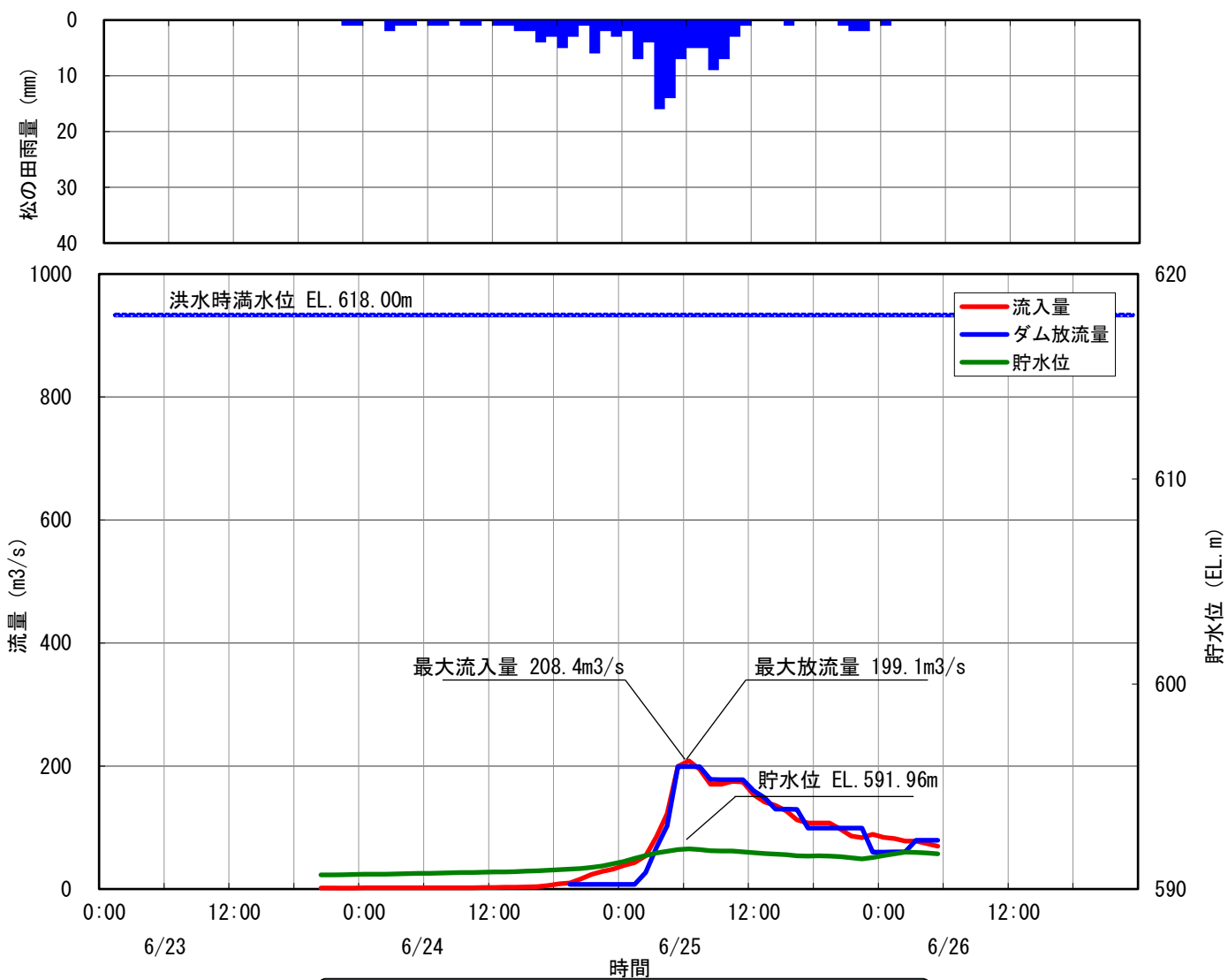
10 小渋ダム洪水調節図 昭和52年6月25日洪水
