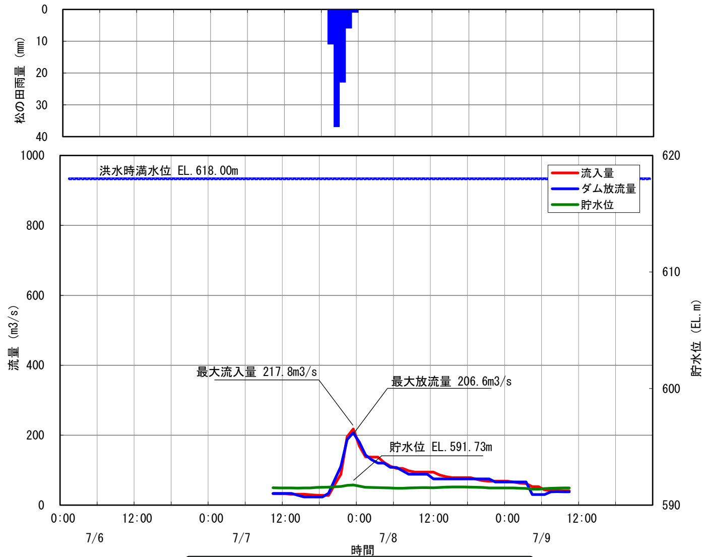
9 小渋ダム洪水調節図 昭和50年7月7日洪水
