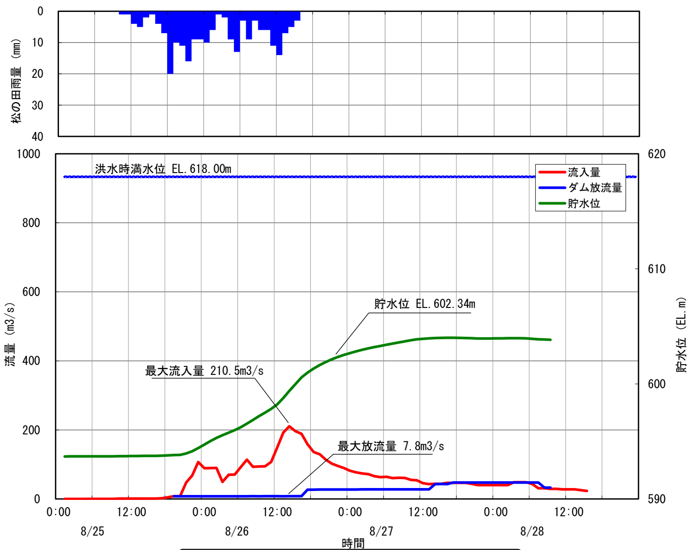
7 小渋ダム洪水調節図 昭和49年8月26日洪水
