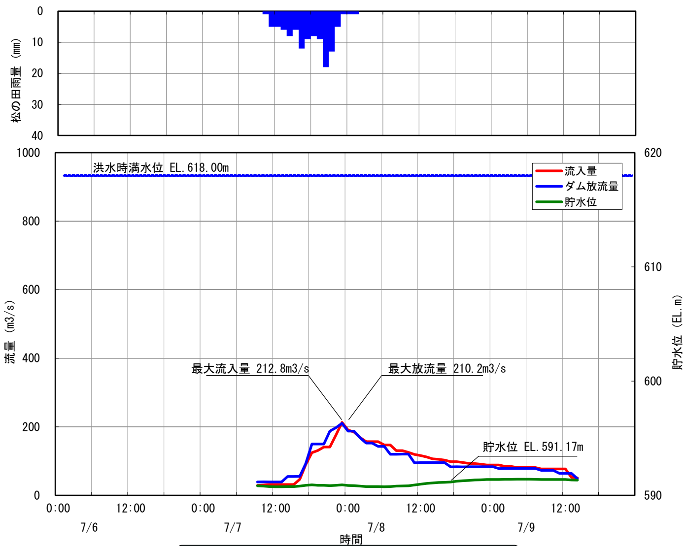
6 小渋ダム洪水調節図 昭和49年7月7日洪水
