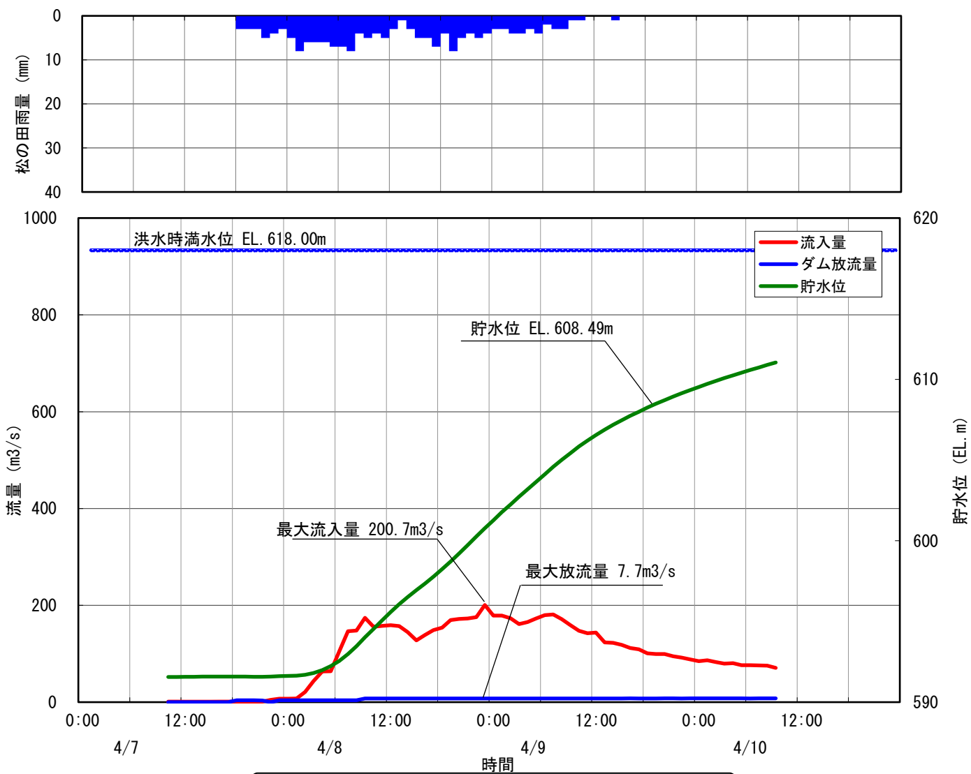
5 小渋ダム洪水調節図 昭和49年4月8日洪水
