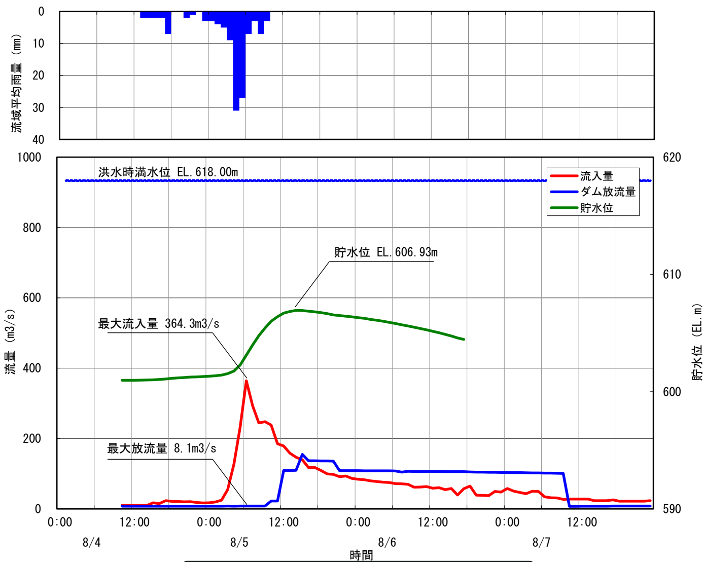
2 小渋ダム洪水調節図 昭和44年8月5日洪水
