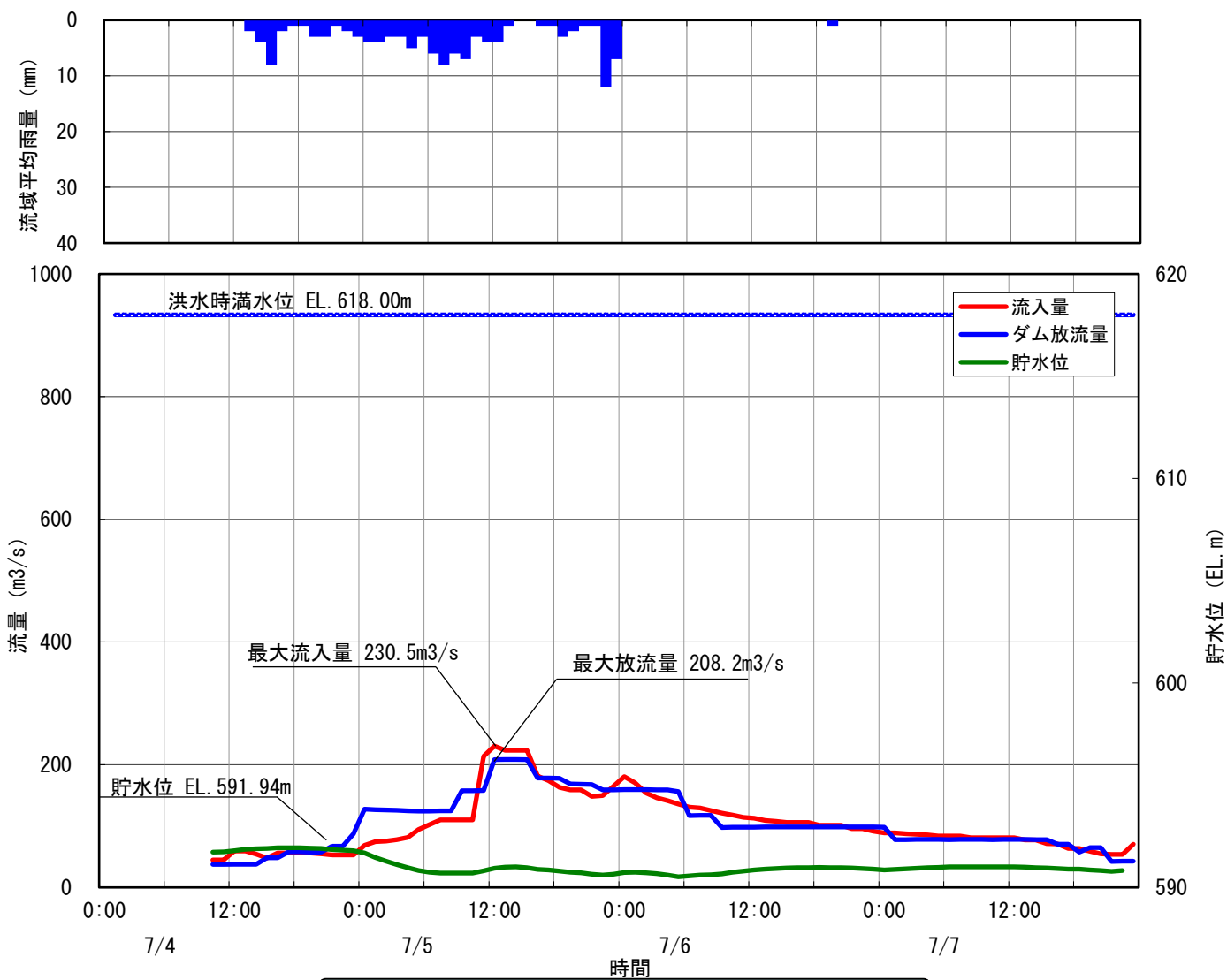
① 小渋ダム洪水調節図 昭和44年7月5日洪水
