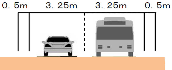
標準断面図
