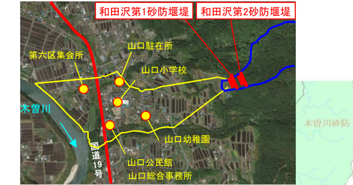
2.和田沢砂防堰堤（中津川市）
