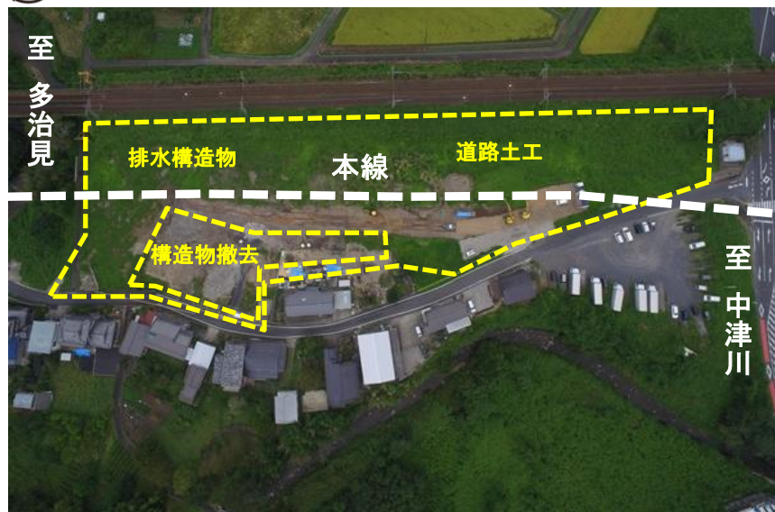
R7.町屋地区道路建設工事
