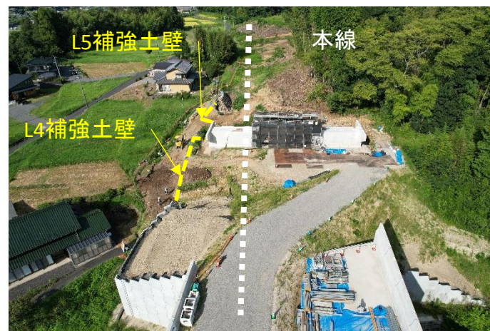
R7.早曾洞地区整備工事
