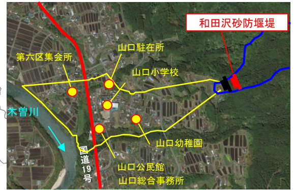
1.和田沢砂防堰堤(中津川市)
