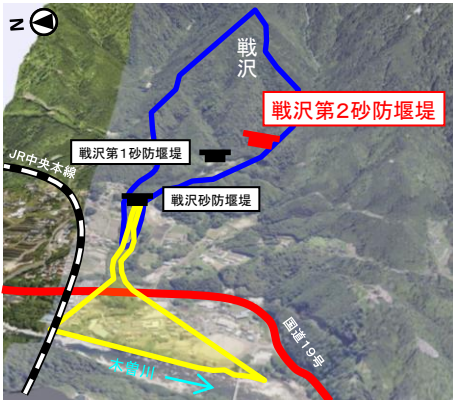
13.戦沢第2砂防堰堤(南木曾町)
