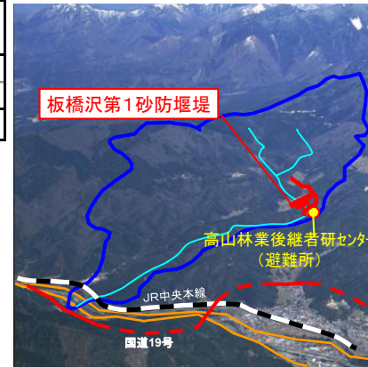
1.板橋沢第1砂防堰堤(上松町)
