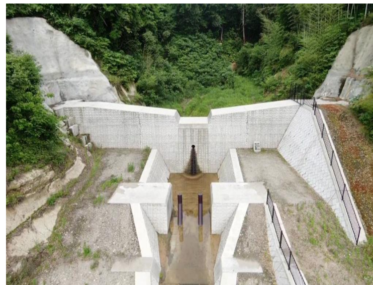
<一の洞第2砂防堰堤と下流の保全対象>
