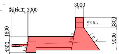
砂防堰堤横断面図
