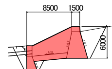
谷止工横断面図
