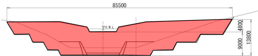
砂防堰堤正面図
