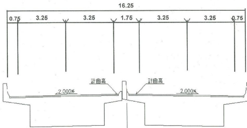
図 2-3 道路構造の概要
